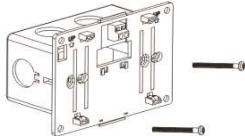
Монтирайте винтовете
